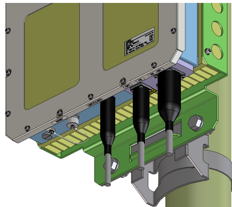
3,5GHz ODU
